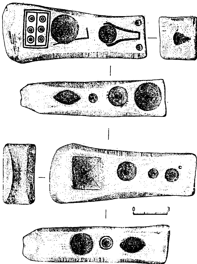
Fig. 6. Matriță din os pentru produs prin presare obiecte vestimentare, descoperită la Costești-Iași.
